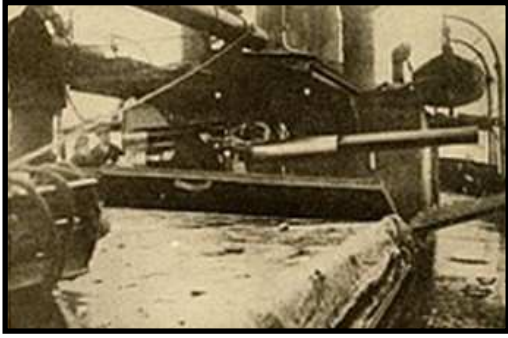
Links: kanonnen op Q-schepen waren weggestopt achter beweegbare of draaibare panelen. Rechts: HMS Tamarisk
