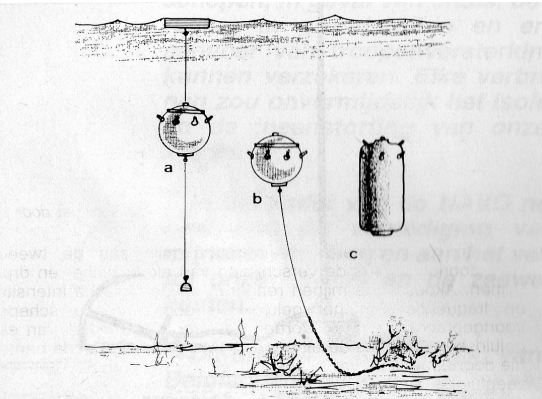
Vrij drijvende mijnen : drijvende mijn met vlotter (a), kruipende mijn (b) en oscillerende mijn (c).
