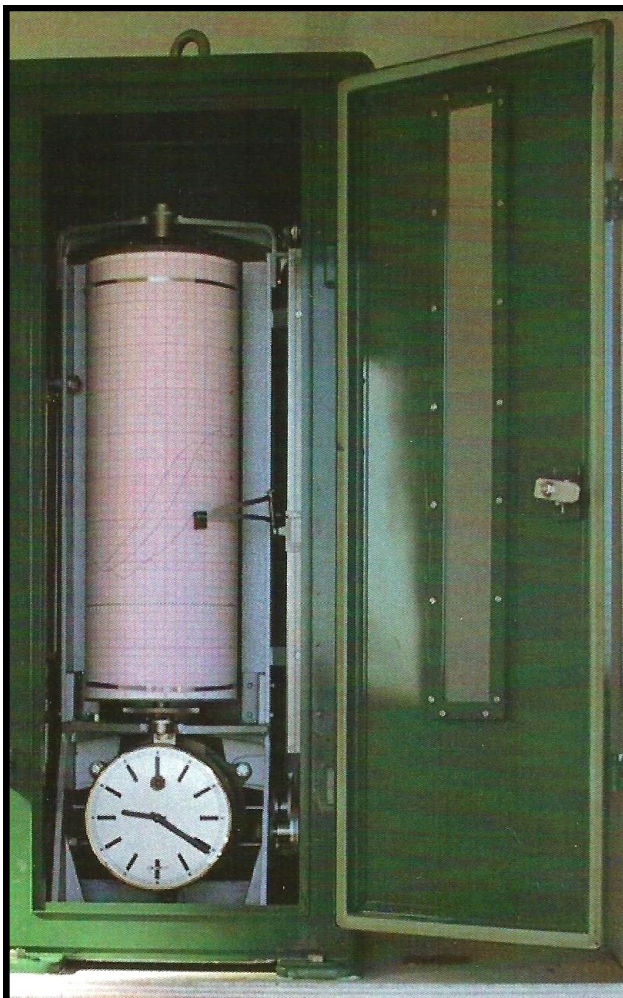
Tijmeter OTT type 20.030
