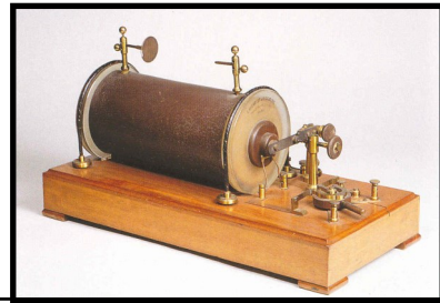
Inductieklos van Ruhmkorff
